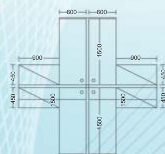
MAX 2 W 3060 x D 3060 x H 1200
